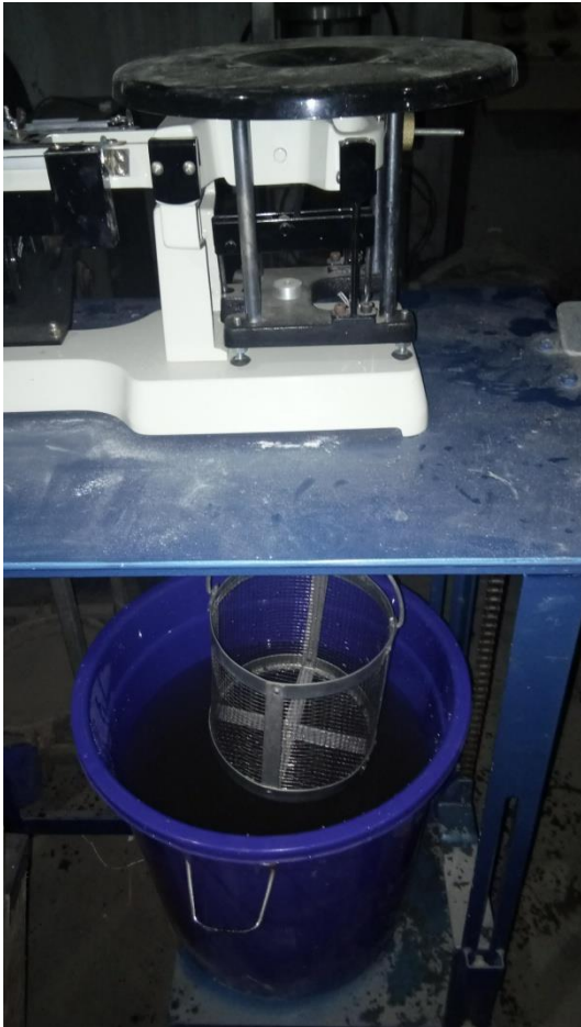
Alat Uji Berat Jenis Kerikil
