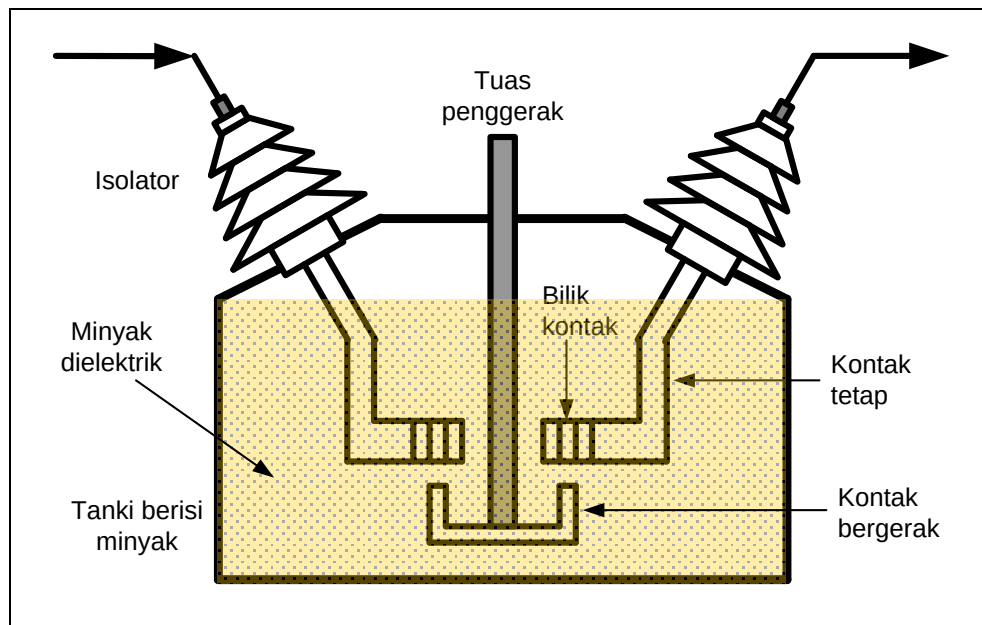
Lampiran 3. Gambar Konstruksi Pemutus PMT Minyak.
