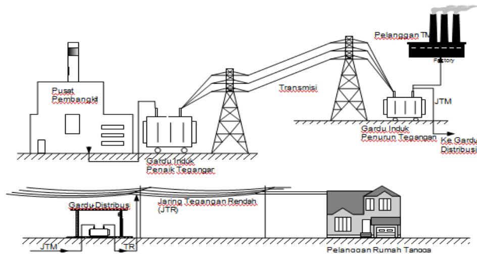
Gambar 2.2 Skema Penyaluran Energi Listrik Dimulai dari Pusat Pembangkit sampai dengan Pelanggan
