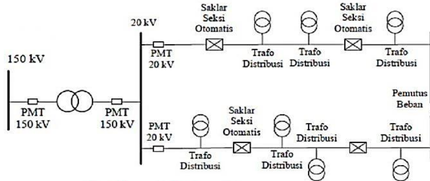
Gambar 2.6 Konfigurasi Jaringan Loop
