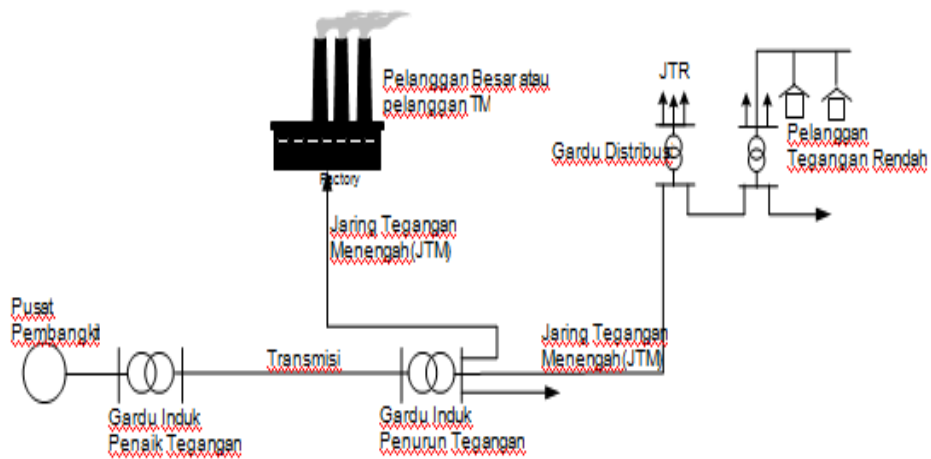
Gambar 2.3 Diagram Satu Garis Penyaluran Energi Listrik Dimulai dari Pusat Pembangkit sampai dengan Pelanggan 1
